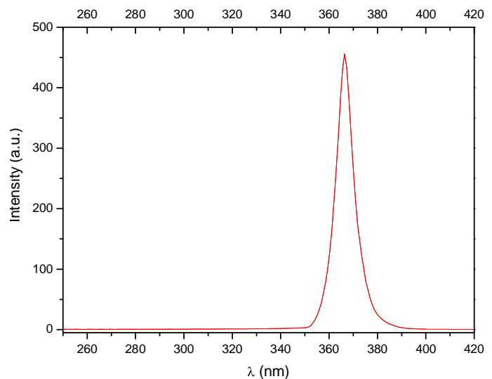
Spektrale Emissionsverteilung von: Blackline-SH
