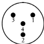
XLR - mini
